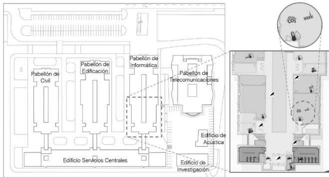
Fig. 1. Plano de la EPCC, y ejemplo de distribución de los sensores en uno de los pabellones.
