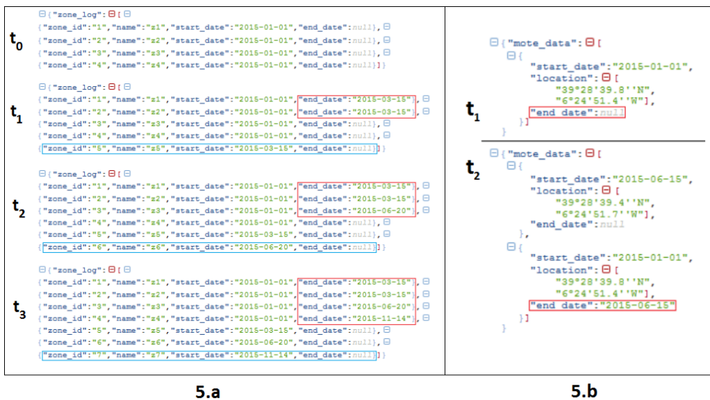
Fig. 5. a) Histórico de las localizaciones geográficas de un datalogger en el tiempo. b) Histórico de las localizaciones geográficas de un datalogger en el tiempo.
