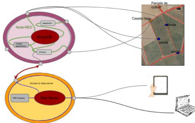
Fig. 1. Esquema de la arquitectura de la plataforma.
