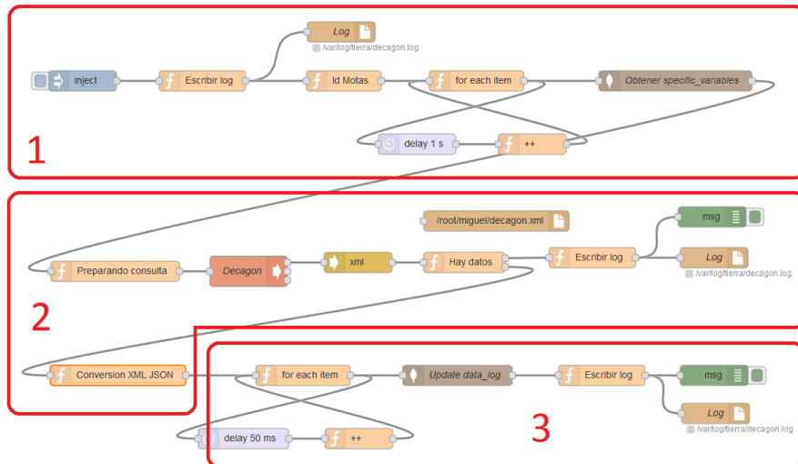
Fig. 3. Estructura del evento de flujo.
