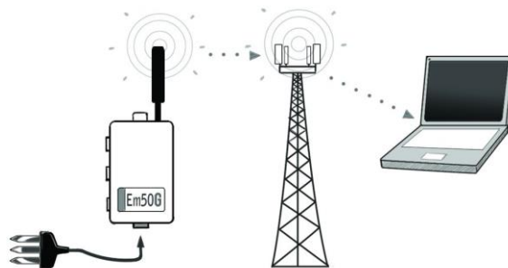
Fig. 2. Esquema de comunicación del datalogger.
